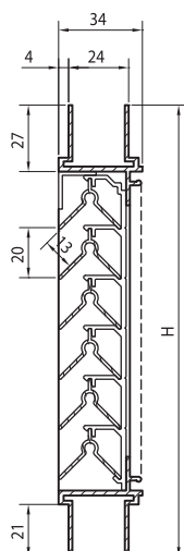
Doorsnedetekening
