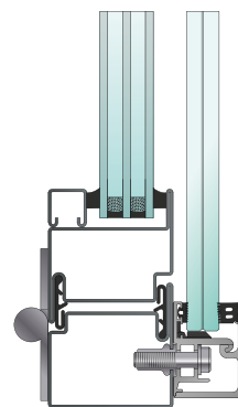
staal kozijn
