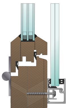
houten kozijn
