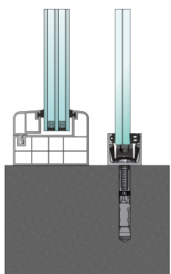
Betonkozijn
