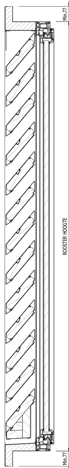
DOORSNEDE A-A
