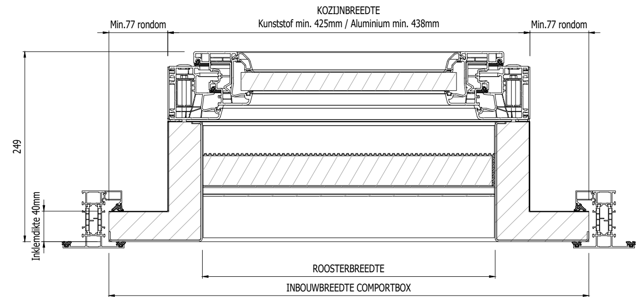
DOORSNEDE B-B
