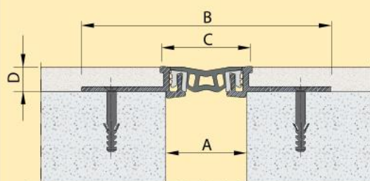
Profiel GFS 40.5
