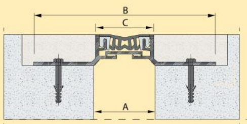
Profiel GFT 50.30
