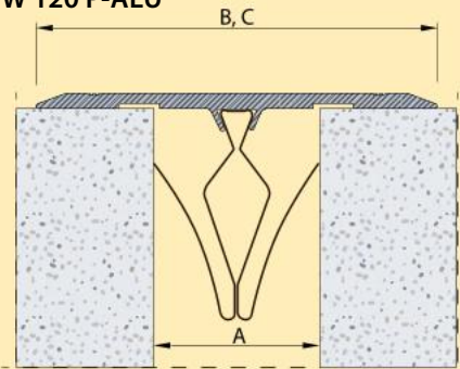
Profiel W 120 P-ALU
