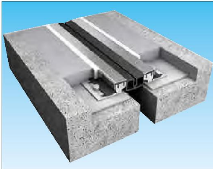
Profiel PDSW 50/30
