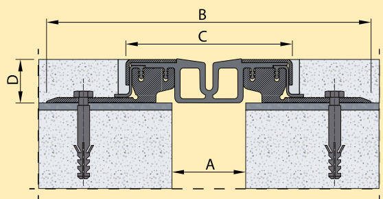
Profiel PDS 50/30
