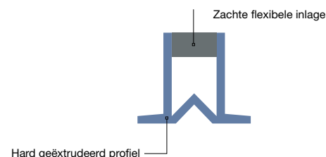
Profiel JF 10/43 (brede profielflenzen)
