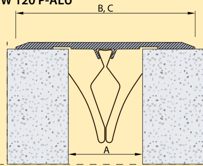
Profiel W 120 P-ALU
