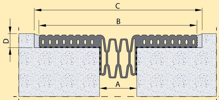
Profiel ZB 100
