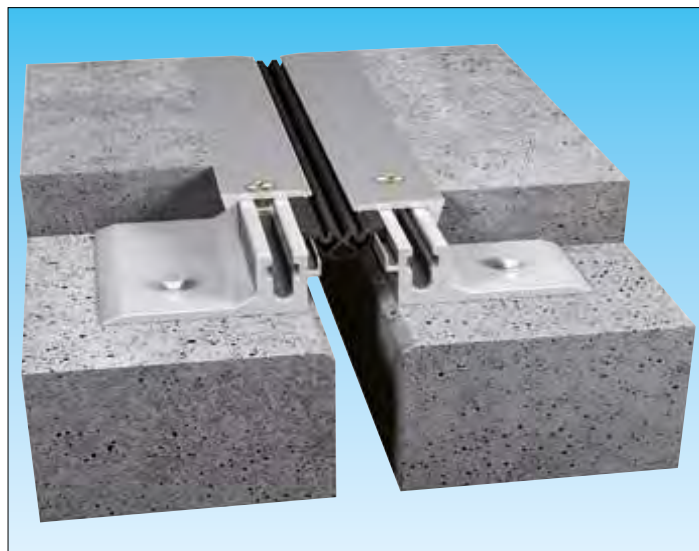
Profiel GFT 40
