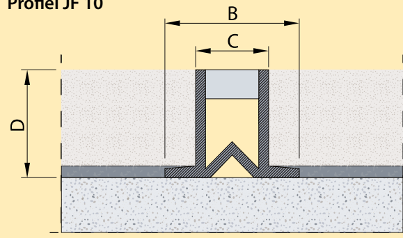
Profiel JF 10
