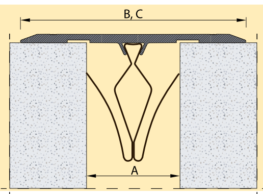
Profiel W 120 P
