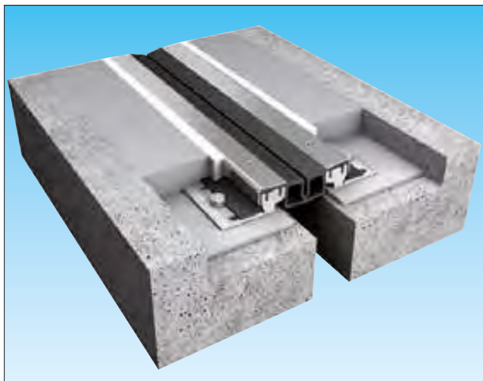
Profiel PDS 50/30
