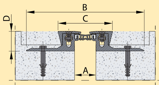
Profiel GFT 40 HD
