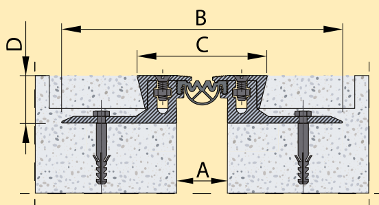
Profiel GFT 40
