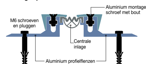
Profiel GFT 40 HD
