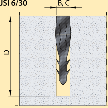
Profiel JSI 6/30
