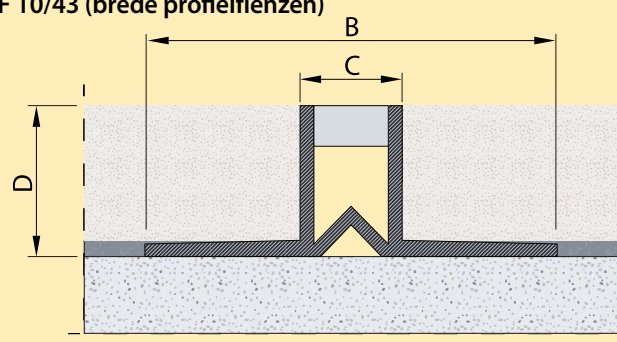
Profiel JF 10/43 (brede profielflenzen)
