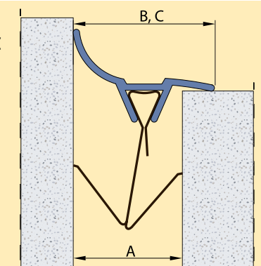
Profiel W 50 A-PVC
