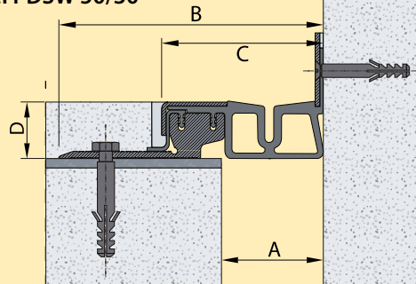
Profiel PDSW 50/30
